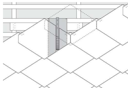
Střešní hák u kosočtvercového krytí 40 × 44 cm
