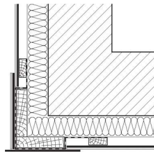
S přesahem desek jako ostrý štít
