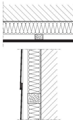
Svislé nosné laťování na vodorovném základním laťování
