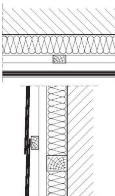
Vodorovné základní laťování, svislé mezilehlé laťování a vodorovné nosné laťování
