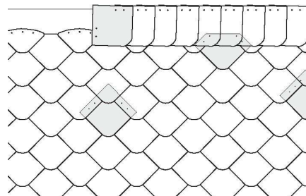
Horní ukončení se stojatou ukončovací řadou a vybiňajícím štítem
