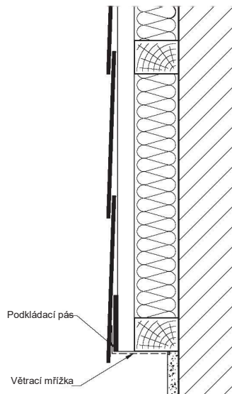
Spodní ukončení u svislého nosného laťování na vodorovném kontralaťování
