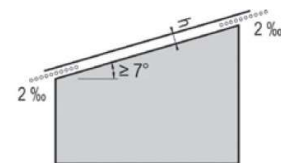
Větrací průřezy u pultových střech
