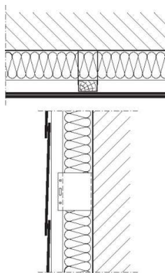
Hliníkový držák tvaru U se svislým nosným laťováním
