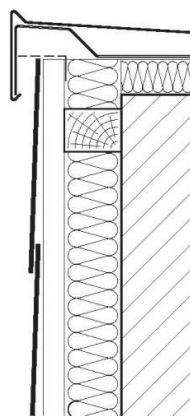
Horní ukončení u atikového krytí
