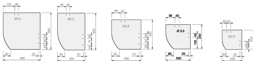
40 × 40 cm, obloukový řez
