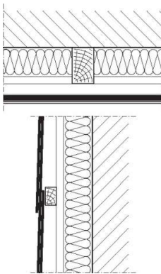
Vodorovné nosné laťování na svislém základním laťování
