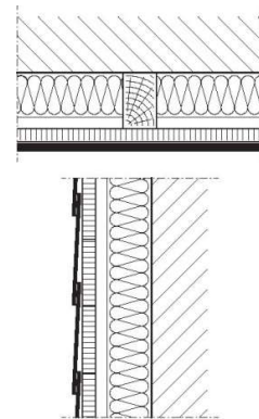
Bednění na svislém základním laťování
