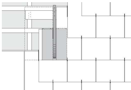
Střešní hák u dvojitého krytí 32 × 60 cm
