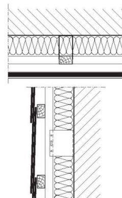
Hliníkový držák tvaru U se svislým základním laťováním a vodorovným nosným laťováním
